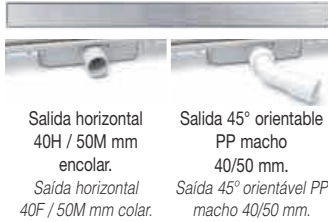
Salida horizontal 40H / 50M mm encolar. Saída horizontal 40F / 50M mm colar.
