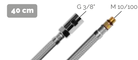
Conexión G 3/8" de 40 cm para modelo 8191 Boquilla M 10/100 de 18 mm longitud x hembra G 3/8" Hose G 3/8" 40 cm length for model 8191 18 mm length M 10/100 nozzle x G 3/8" REF. 45941 · PVP: 15,86 €
