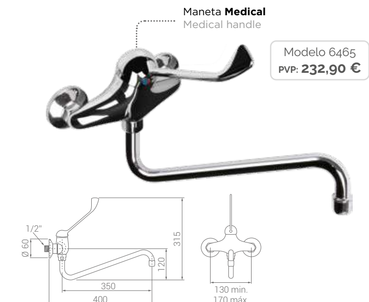
Monomando con caño bajo de 350 mm Mixing faucet with 350 mm low spout
