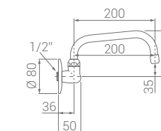
Caño giratorio recto de 300 mm 300 mm straight rotating spout
