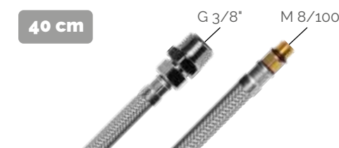
Conexión G 3/8" de 40 cm para modelo 8195 Boquilla M 8/100 de 18 mm longitud x macho G 3/8" Hose G 3/8" 40 cm length for model 8195 18 mm length M 8/100 nozzle x G 3/8" REF. 45971 · PVP: 13,99 €
