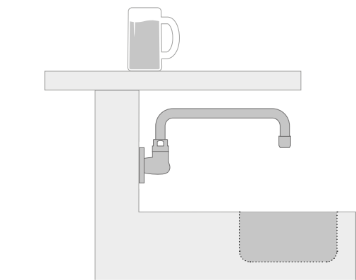
Caño giratorio recto de 250 mm 250 mm straight rotating spout
