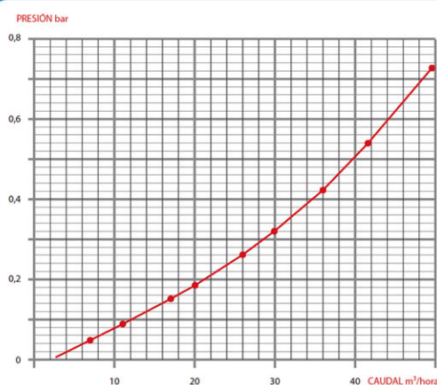
PÉRDIDA DE CARGA DE EQUIPOS NOVHIDRO AUTO 3" L-BER
