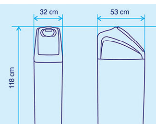
Dimensiones FLAMINGO C25-C38
