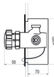
Con válvula de vaciado y conducto guía
